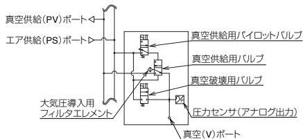
空気圧回路図 [搭載ユニット1台分]
