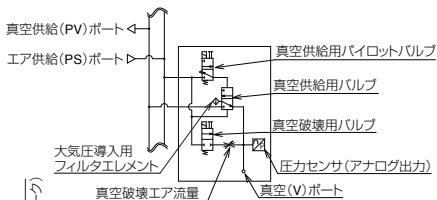
空気圧回路図 [搭載ユニット1台分]
